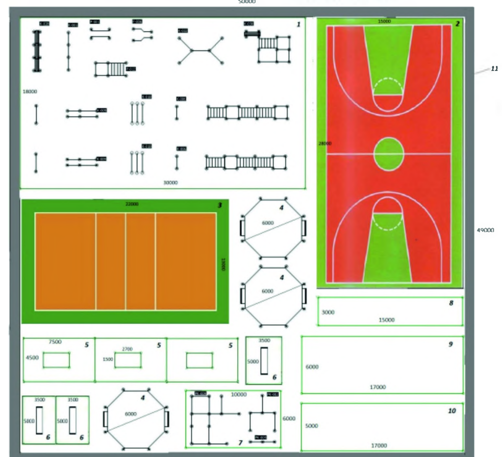
11 СПОРТИВНЫЙ ПАРК РАЗМЕРОМ 50/49 М С ПОКРЫТИЕМ ИЗ РЕЗИНОВОЙ КРОШКИ И ТРОТУАРНОЙ ПЛИТКИ
