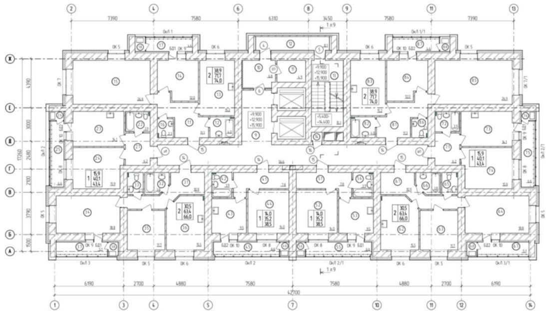
План 5-го - 7-го этажей
