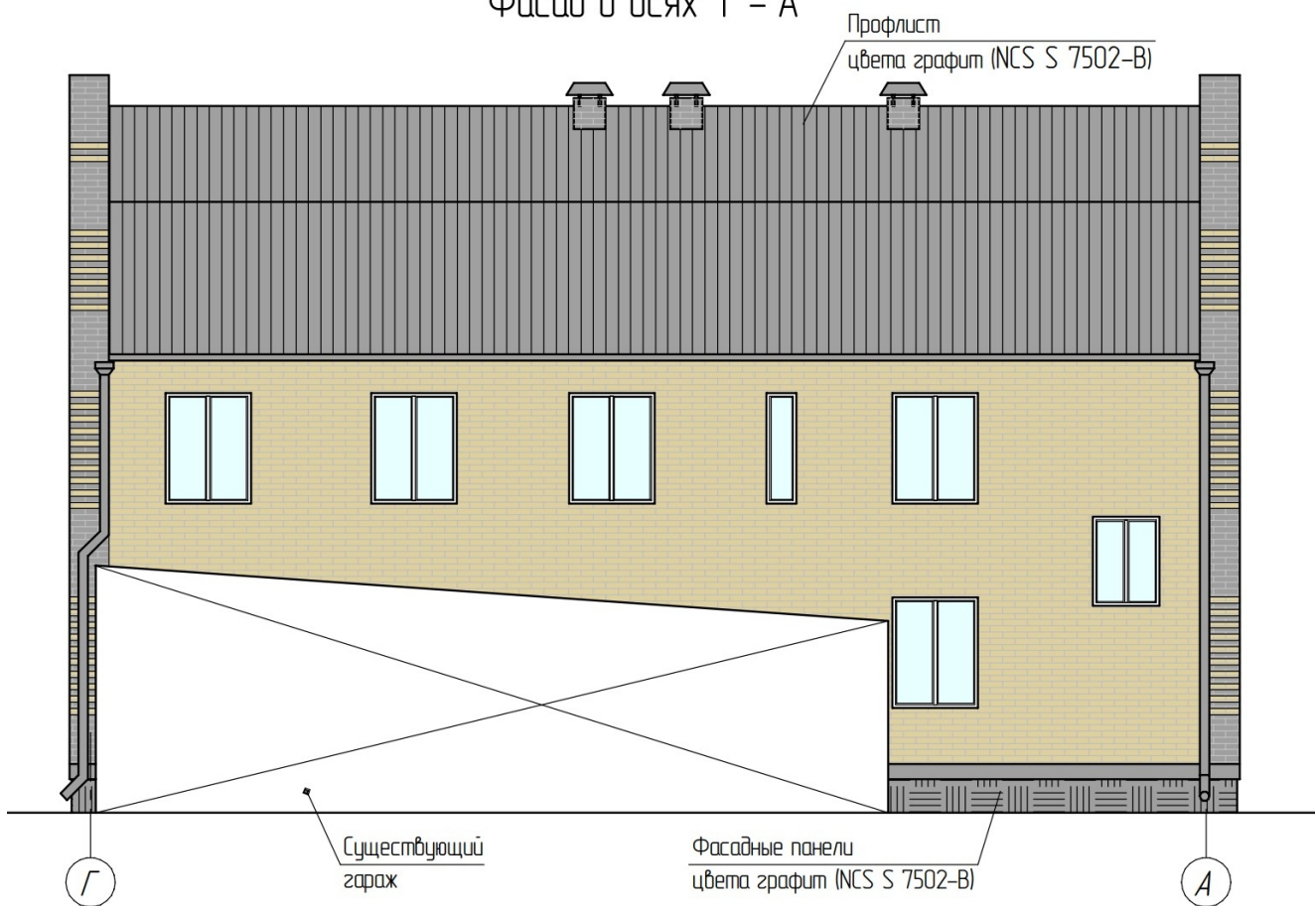
Фасад в осях "Г"-"А"
