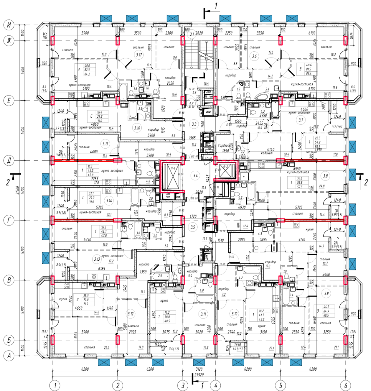
План 3-16-го этажей
