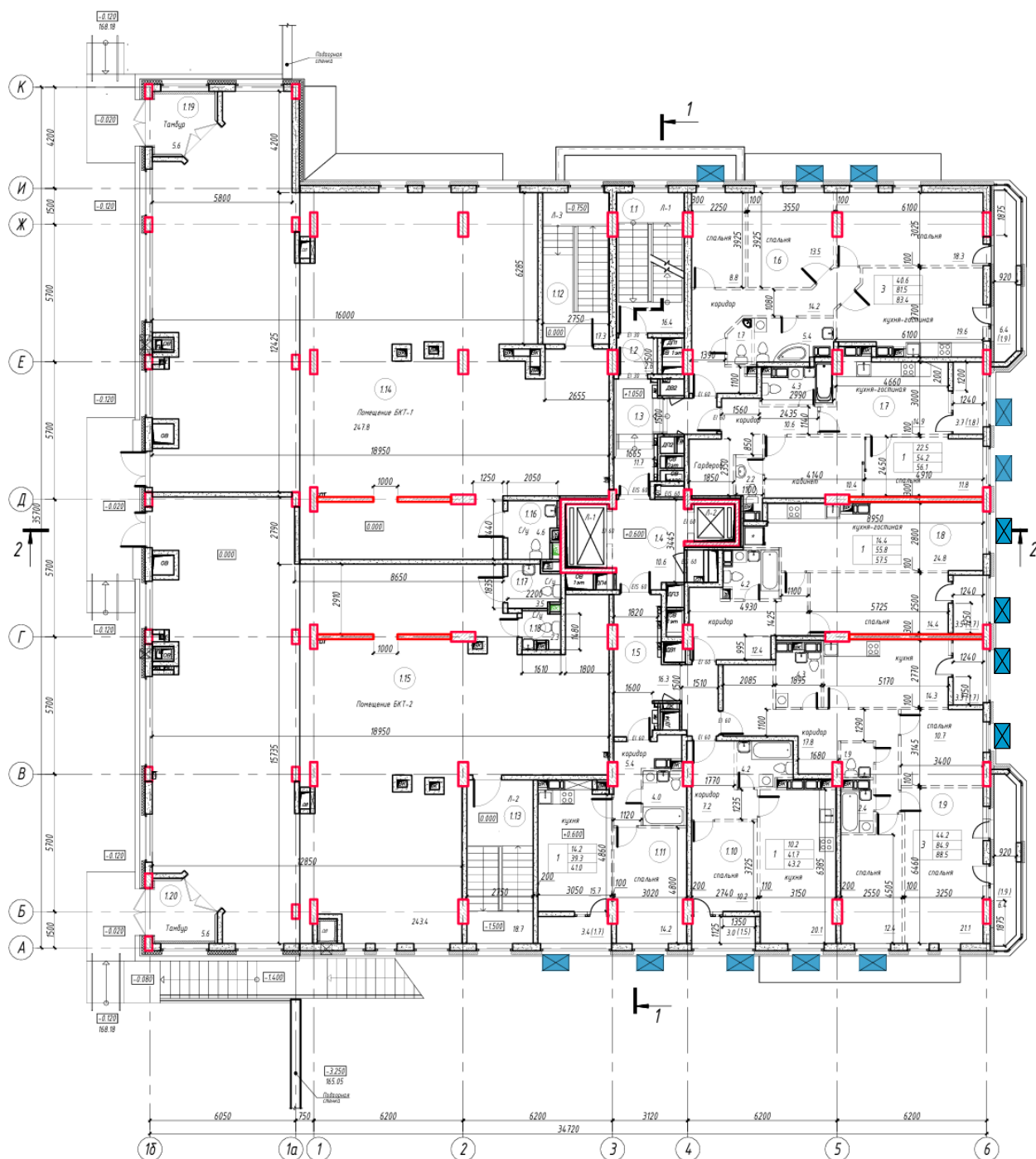
План 1-го этажа
