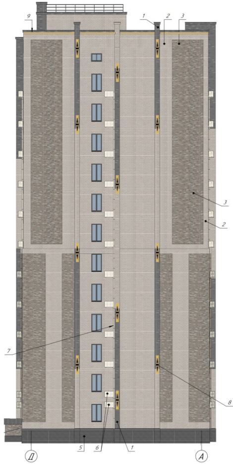
Фасад в осях "II" - "А"
