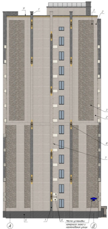
Фасад в осях "А" - "Д"
