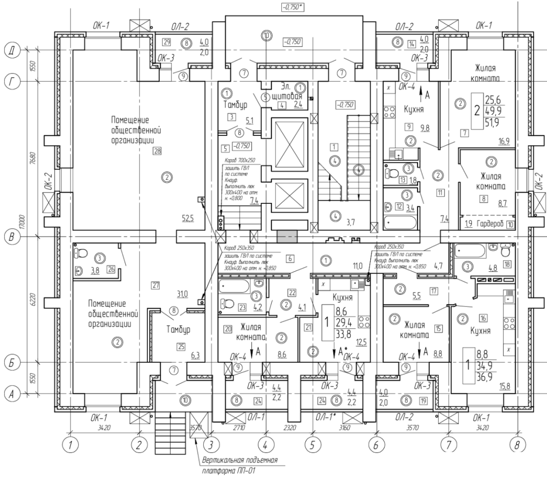
План 2-6го этажа
