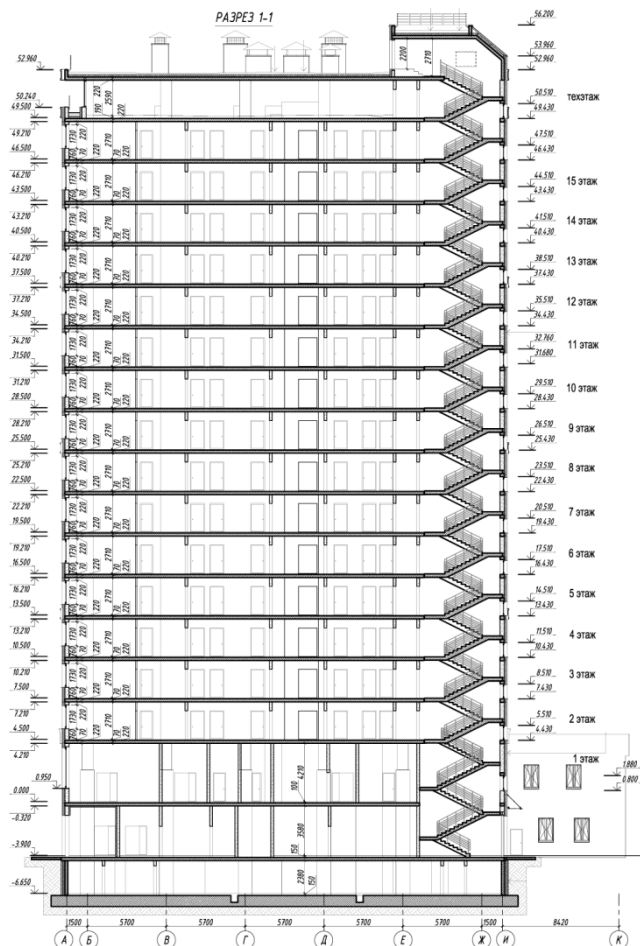
РАЗРЕЗ 1-1
