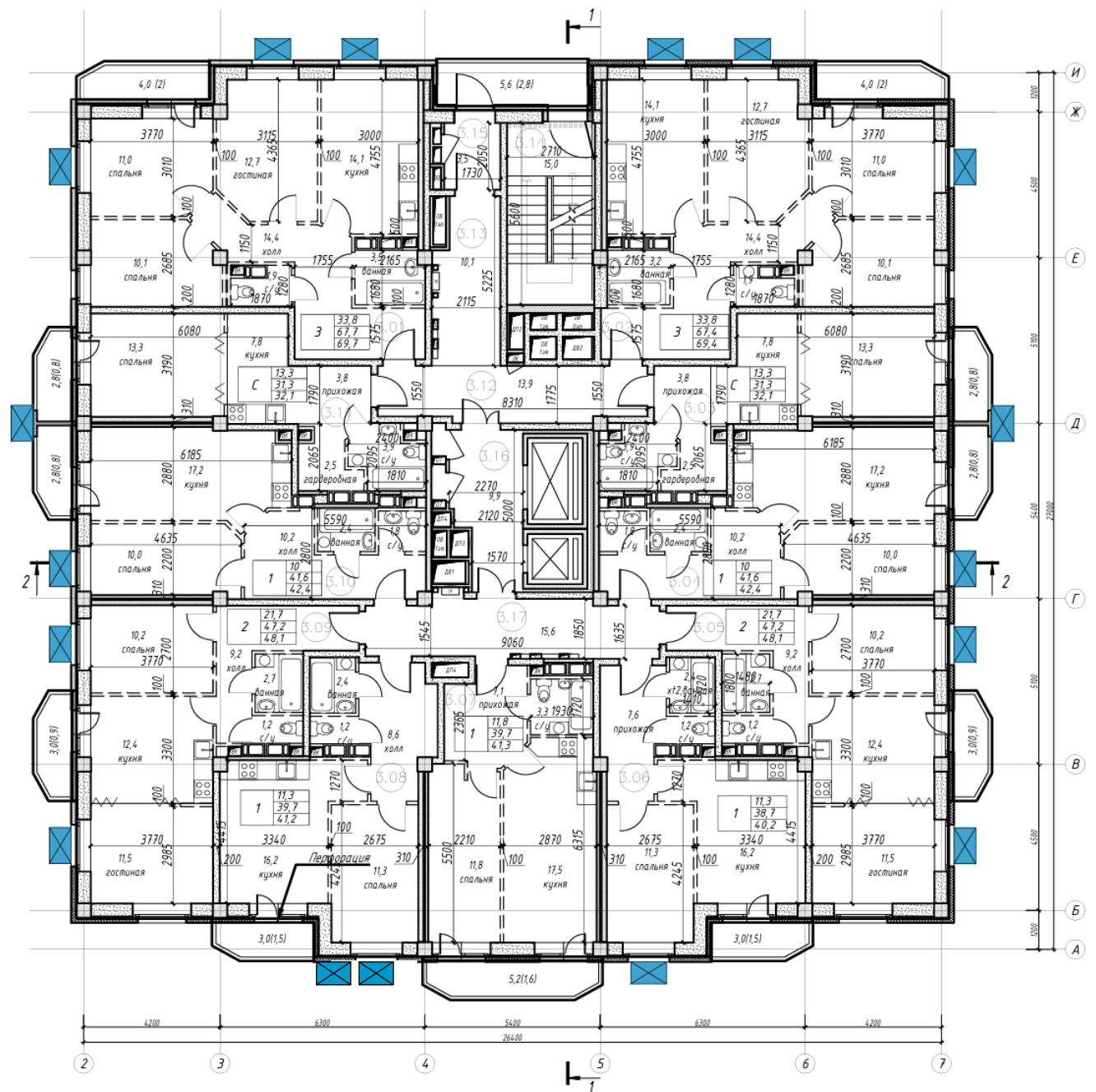
План 3-16-го этажей
