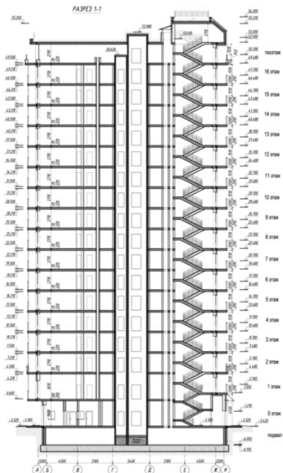
РАЗРЕЗ 1-1
