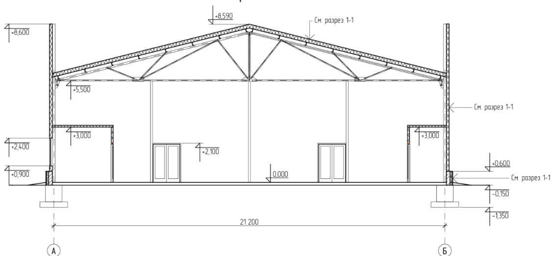
Разрез 2-2
