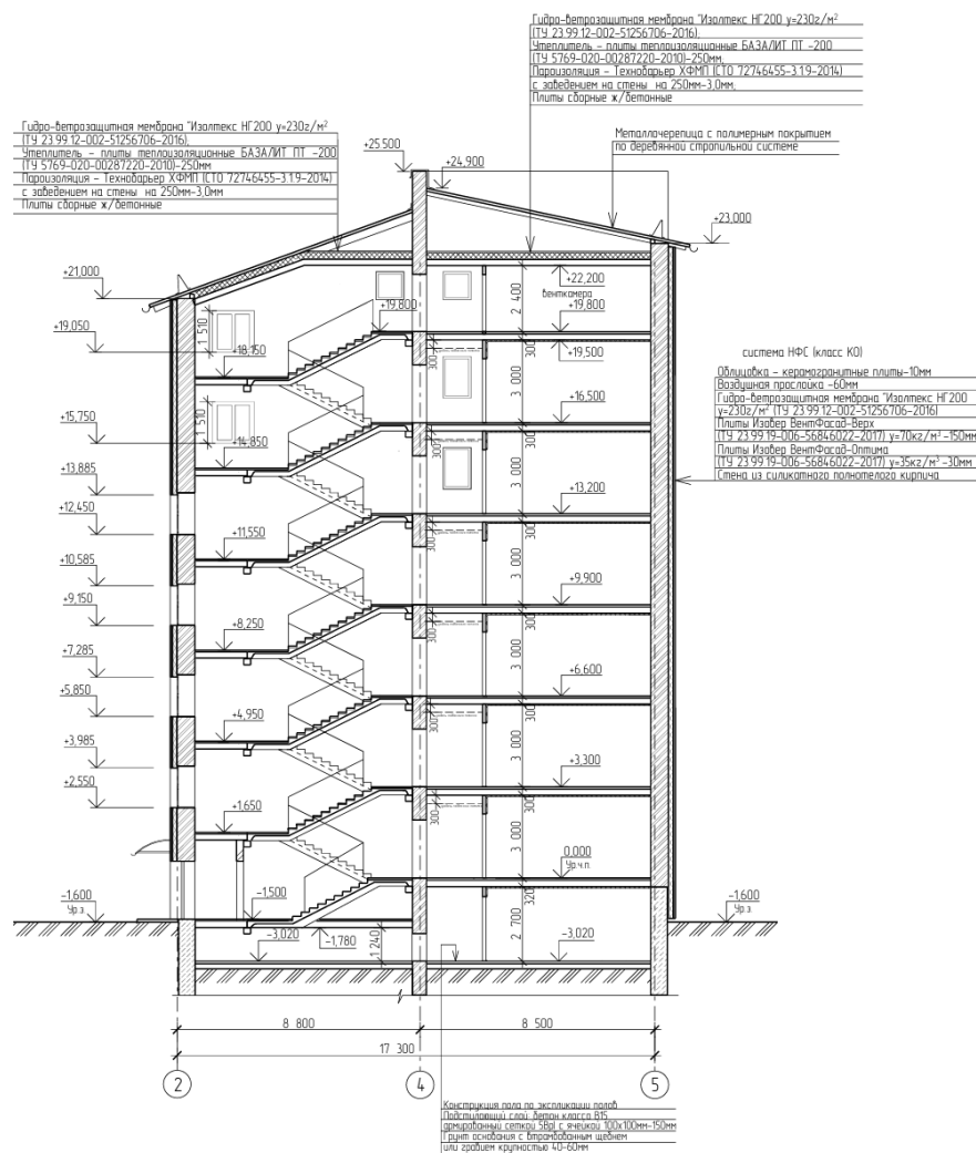
Разрез 1-1
